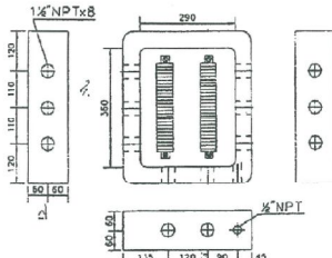
附廠式組合端子板 2.5mm 2 x 37P x NYLON
