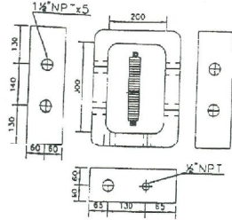
附廠式組合端子板 2.5mm 2 x 37P x NYLON
