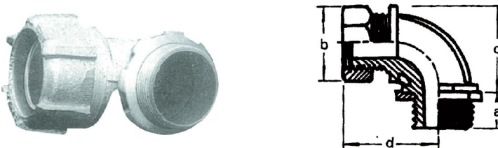
90° 彎外牙軟管接頭 CFC TYPE
